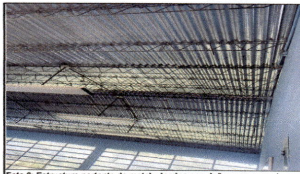
Foto 6: Estructura portante de metal y lamina con daños por corrosión.
